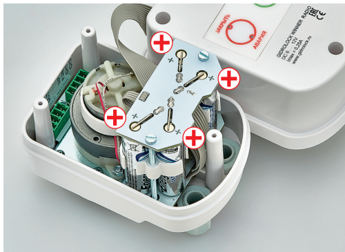
Фото 16. Электропривод со снятой верхней крышкой
