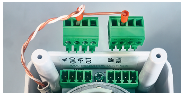
Фото 24. Подключение проводного выключателя
