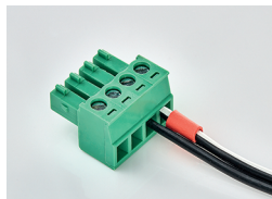
Фото 19. Подключение внешнего блока питания +12 В к ответной части разъема электропривода
