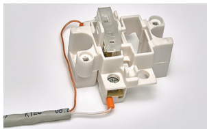
Фото 23. Подключение проводного выключателя
