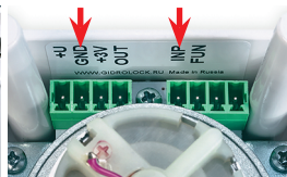
Фото 13. Клеммы подключения проводных датчиков — INP, GND
