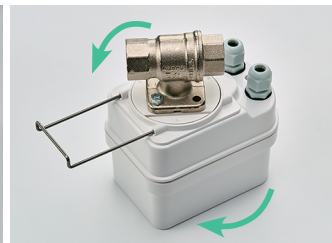
Фото 5. Крепление электропривода к шаровому крану с помощью металлической скобы
