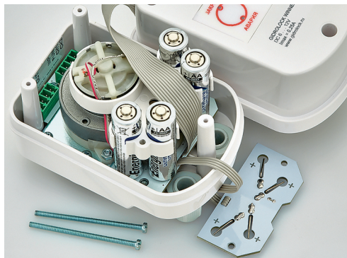
Фото 17. Контактная площадка снята, батарейки могут быть заменены
